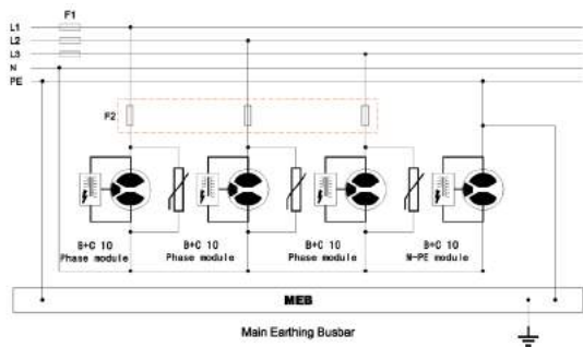
TPS B+C 3P+N 原理图
