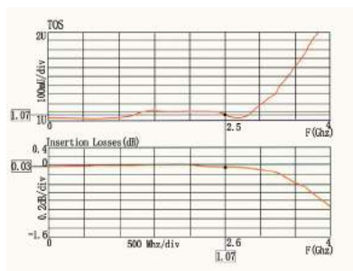
气体放电管保护原理和特性曲线
