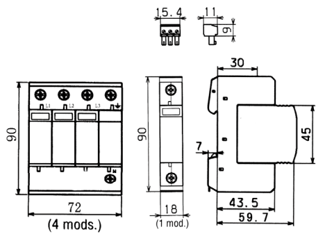
模块及通信端子尺寸图
