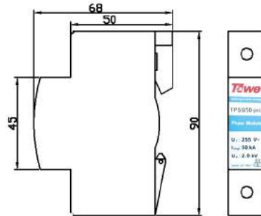
尺寸图
