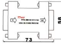
产品尺寸图
