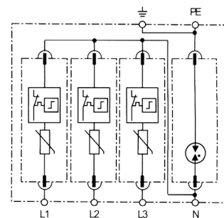
3P+N 原理图
