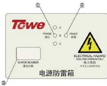
三相电源防雷箱控制面板示意图 (③为选配功能)
