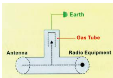
气体放电管保护原理和特性曲线
