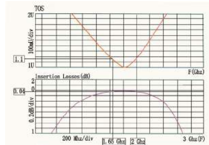
1/4 波长保护原理和特性曲线
