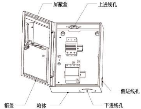
TPS-UN 通用型电源防雷箱内部结构图
