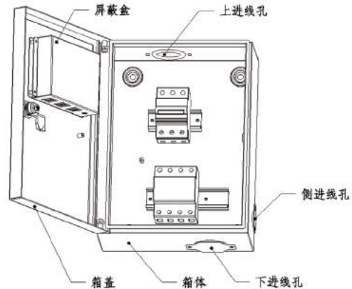
三相电源防雷箱结构图 (电涌保护器和断路器上下安装)
