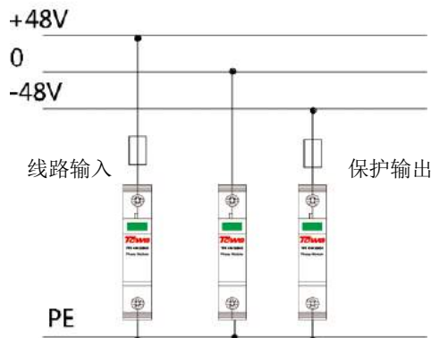
保护电路接线示意图
