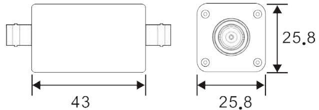
产品尺寸图
