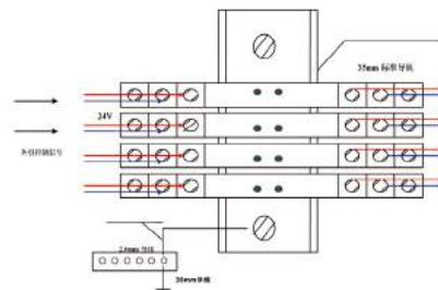
控制信号线电涌保护器安装图
