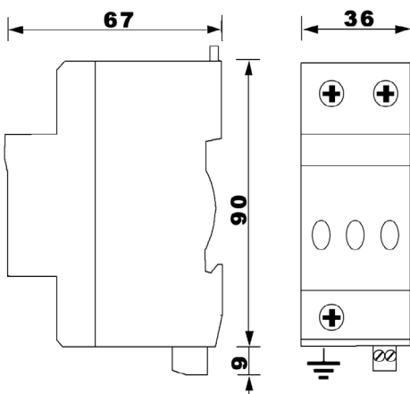
产品尺寸图
