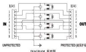
TTS-RJ45-E155/8S, E1000/8S 原理图
