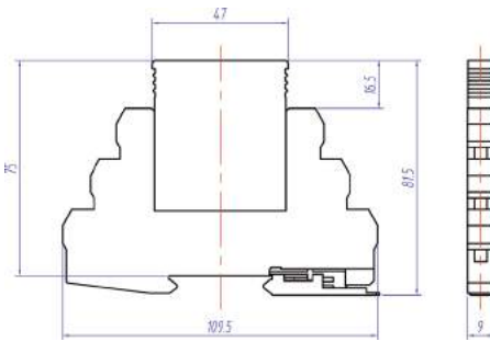
产品尺寸图
