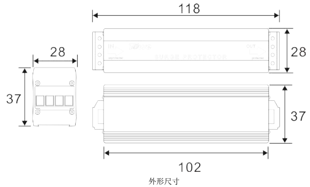
外形尺寸
