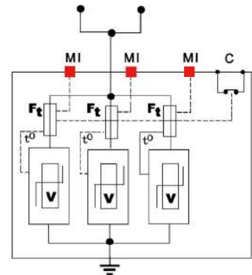
工作原理
