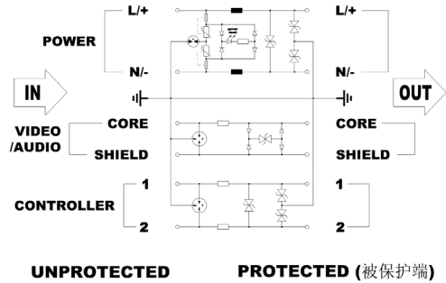
工作原理图
