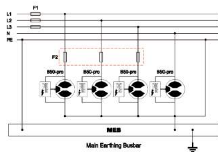
TPS B50-Pro 4P 接线图
