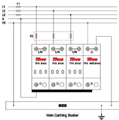
3P+N 接线示意图
