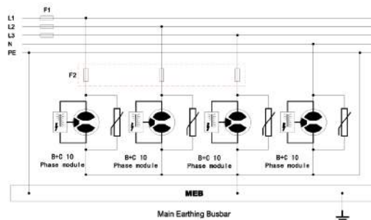
TPS B+C 4P 原理图
