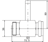
TCS-Q-7/16-50MF-900 尺寸图
