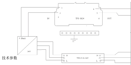
电涌保护器接线图
