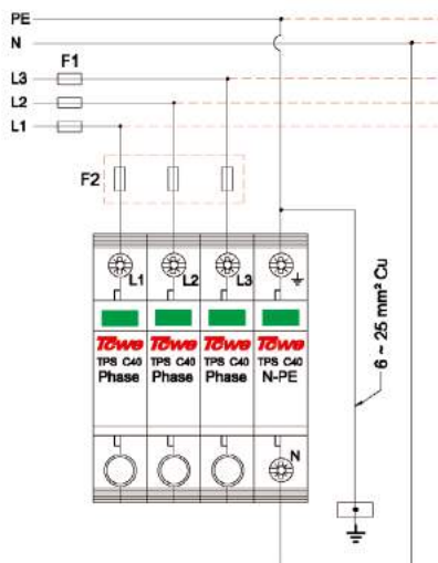
TPS-B65/C40/D20 电涌保护器 3P+N 接线图
