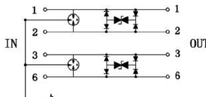
RJ45-E100/4S 产品工作原理图
