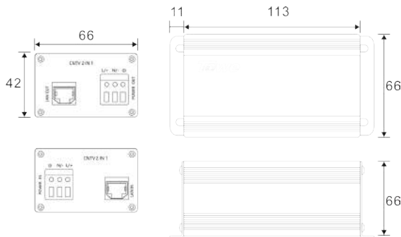
外型尺寸
