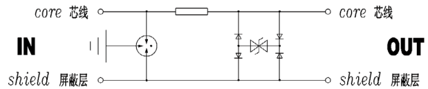
原理图
