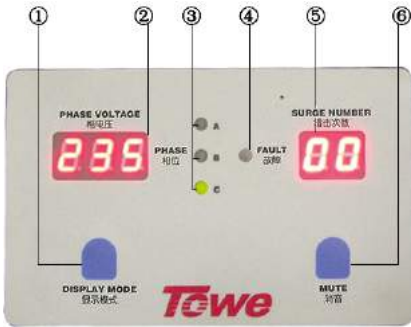
控制面板 ①手动 / 自动电压显示选择键 ②在线电压 (L-N) 显示 ③当前电压相位显示 ④当前故障相位显示 ⑤雷击次数显示 ⑥消音键
