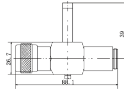
TCS-Q-N-50MF-2400 尺寸图
