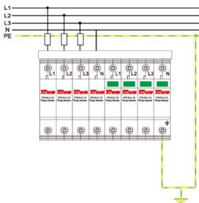
TPS B+C/10 4P 接线图
