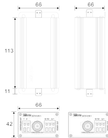
外型尺寸
