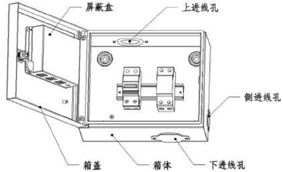
单相电源防雷箱结构图 (电涌保护器和断路器并排安装)
