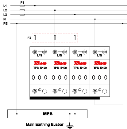
4P 接线示意图
