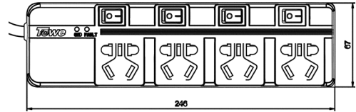
D10 JF4 产品及尺寸图
