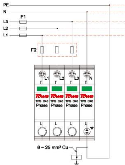
TPS-B65/C40/D20 电涌保护器 4P 接线图
