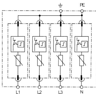
4P 原理图
