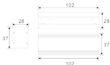
RJ45-E100, E155/4S 尺寸图
