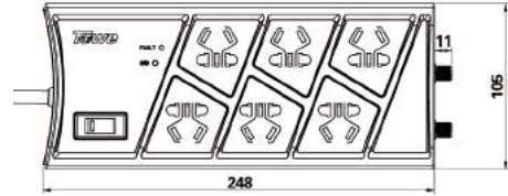
TPS D10 JF6 尺寸图
