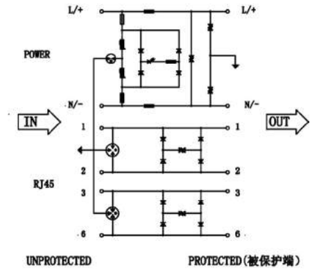
工作原理图
