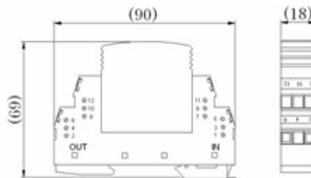
产品尺寸图
