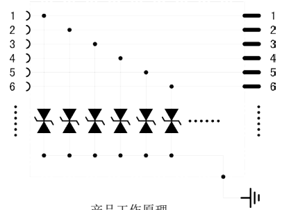
产品工作原理
