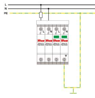
TPS B+C/10 2P 接线图
