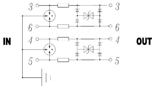
产品工作原理图
