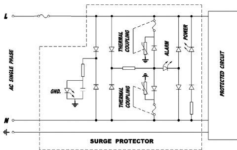
产品原理图
