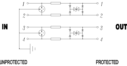
产品工作原理图
