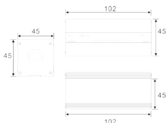
TTS-RJ45-E155/8S, E1000/8S 产品尺寸
