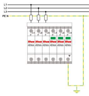
TPS B+C/10 3P 接线图
