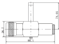
TCS-Q-N-50MF-900 尺寸图
