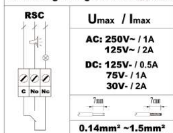
遥信端子接线图
