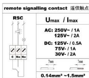
TPS 系列电涌保护器遥信端子接线图
